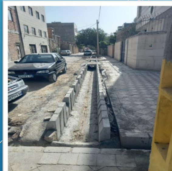
اجرای دال فلزی خیابان امام خمینی
